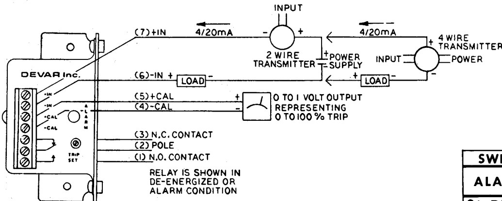
FIG. 1 WIRING DIAGRAM
